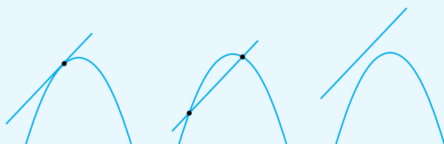
مماس (ریشه مضاعف)
